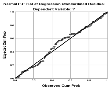
Gambar 1. Uji Normalitas
