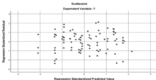
Gambar 2. Uji Heteroskedastisitas
